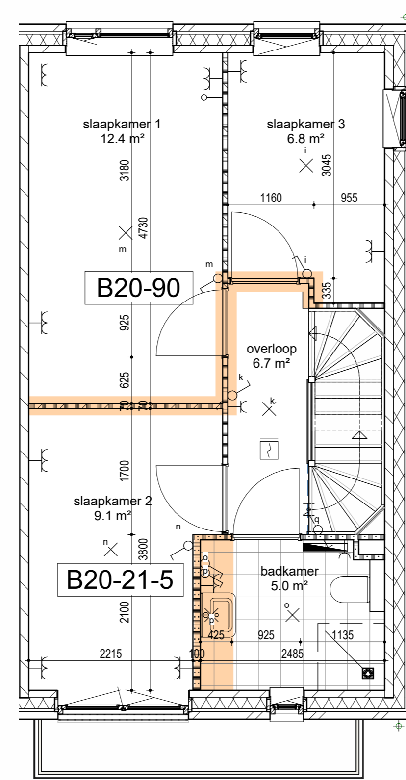
G3/G3s - 1e verdieping
