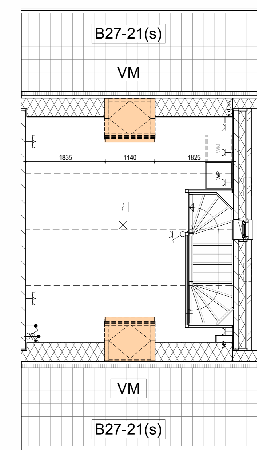
G3/G3s - 2e verdieping
