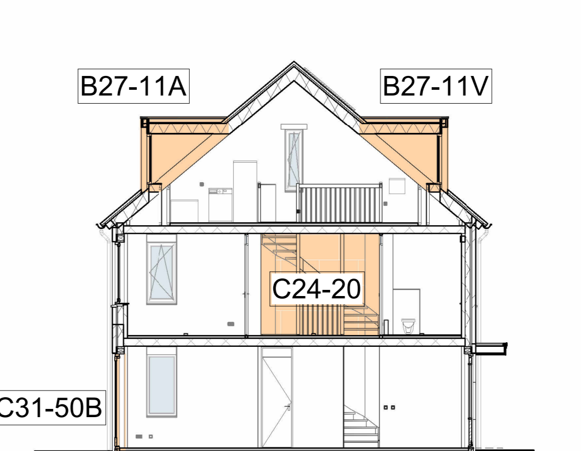
G3/G3s - doorsneden
